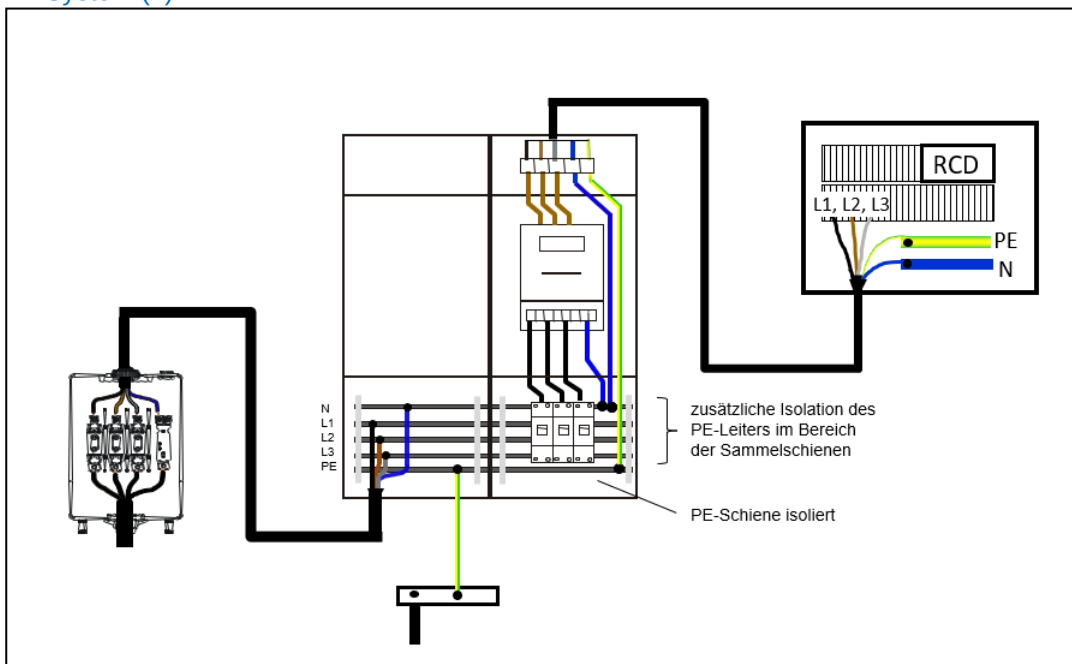
Bild 4 TT-System (2)
