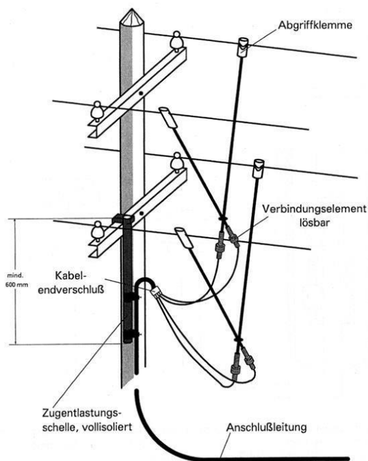
Abbildung: Anchlusselemente für Freileitungsanschluss nach DIN VDE 0680-3
